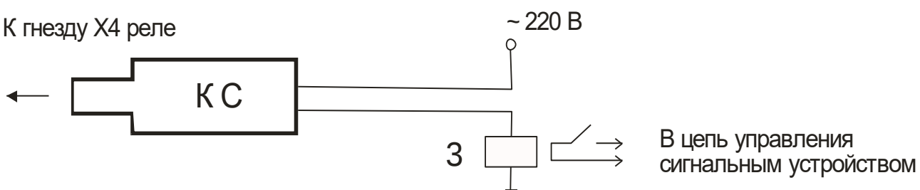
Рисунок 7 - внешний вид и варианты схем подключения контакта сигнального КС:
